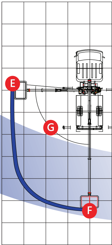
Biểu đồ làm việc (sau) Working range chart (from rear)
