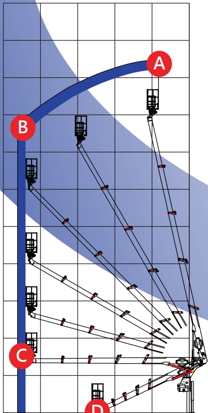
Biểu đồ làm việc (hông) Working range chart (from side)
